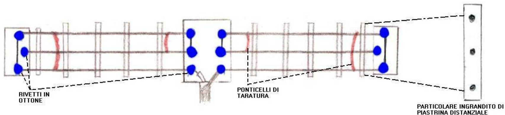
Figura 2. Schema pratico; il materiale utilizzato per costruire gli isolatori e le piastrine è vetroresina spessa 2mm.
